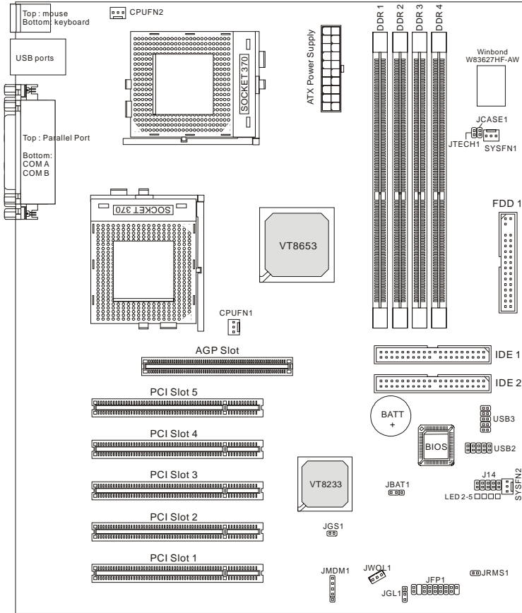
Pro266TD Master (MS-9105) ATX Mainboard
